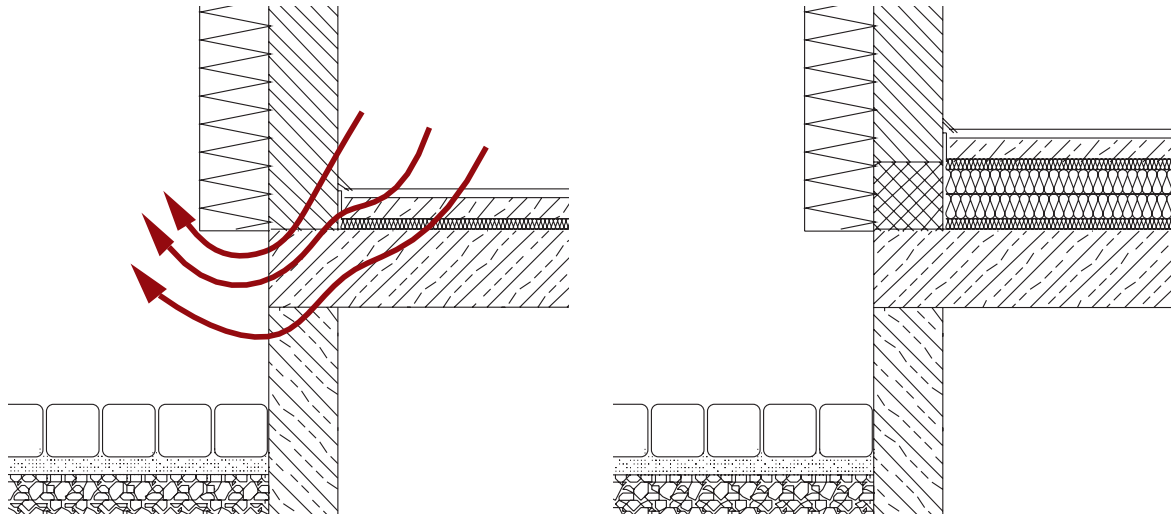
Abbildung 2: Wärmebrücke Kelleranschluss und Sockeldämmung XPS / Schaumglas
