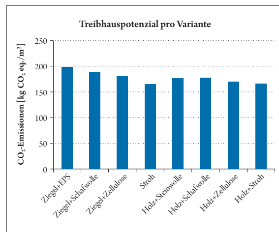
Abbildung 9: Treibhauspotenzial pro Variante
