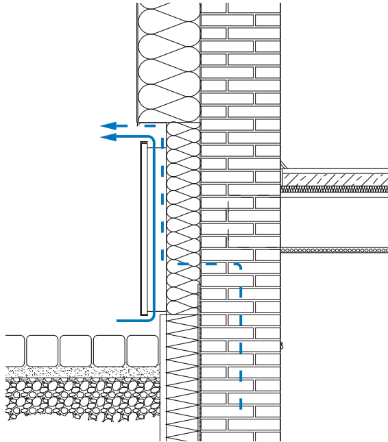
Abbildung 6: Sockelentfeuchtung
